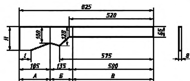
Черт. 5
