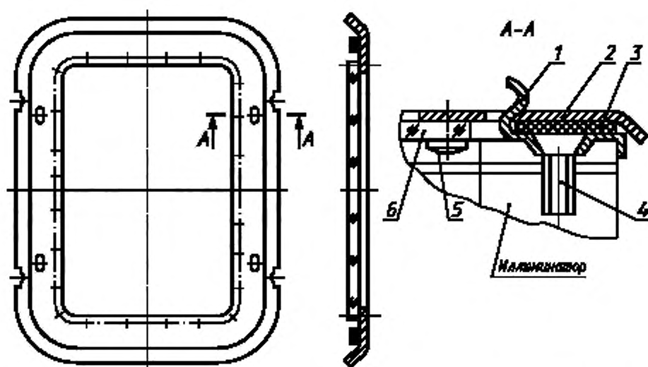
1 — защелка; 2 — рамка щитка; 3 — прокладка; 4 — винт; 5 — заклепка; 6 — органическое цветное стекло
