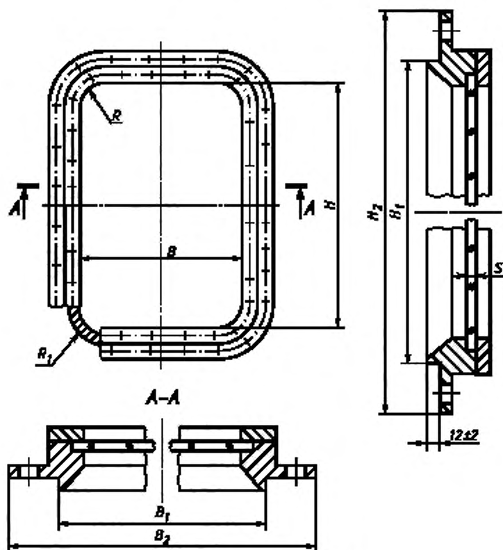
Рисунок 4 — Исполнение NOB
