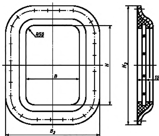
Рисунок 11 — Исполнение NUB
