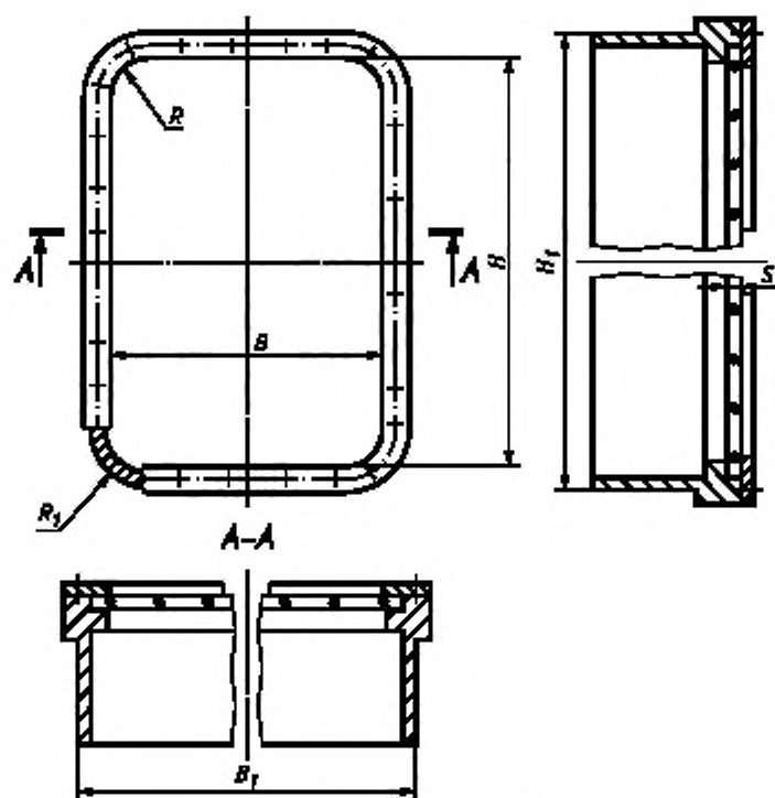
Рисунок 5 — Исполнение NOW
