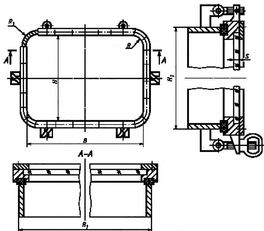
Рисунок 10 — Исполнение JTW
