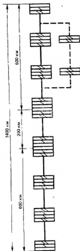
Номинальная цепь канала ТЧ внутризоновой сети
