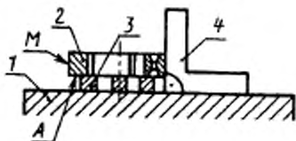
1 — поверочная плита; 2 — сердечник; 3 — опора; 4 — угольник УЛП
