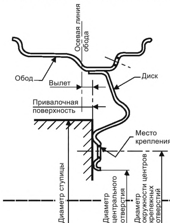
Рисунок 1 — Профиль колеса
