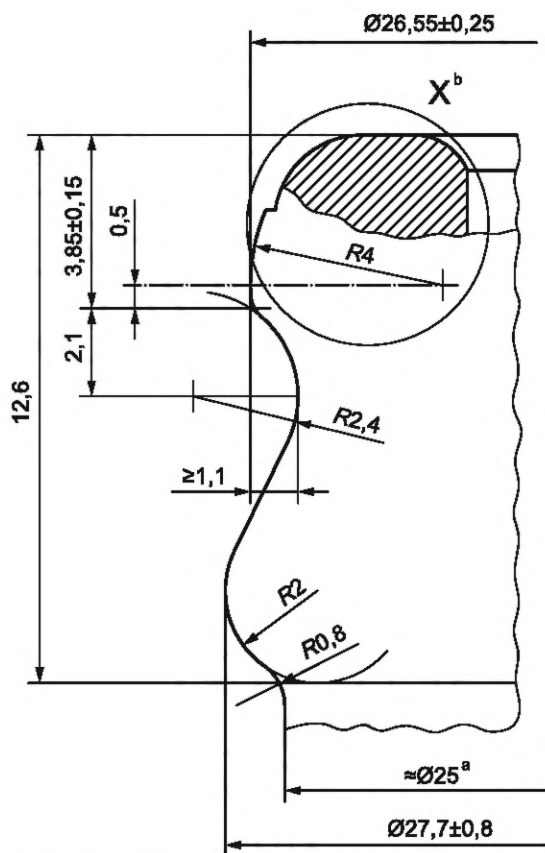
Рисунок 2 — Профиль венчика
