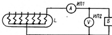
Б—источник напряжения накала; ИП1—амперметр; ИП2—вольтметр; L—индикатор.
