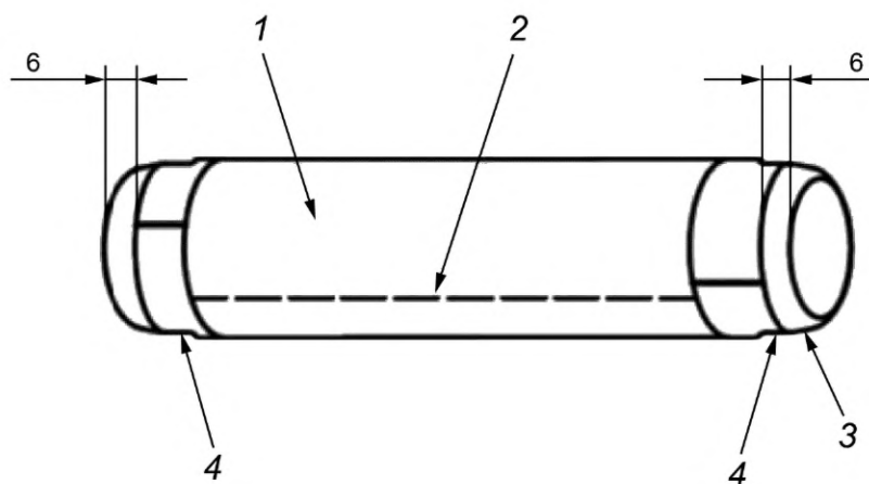
Рисунок 1 — Установка испытуемой пробы на полиуретановой трубке
