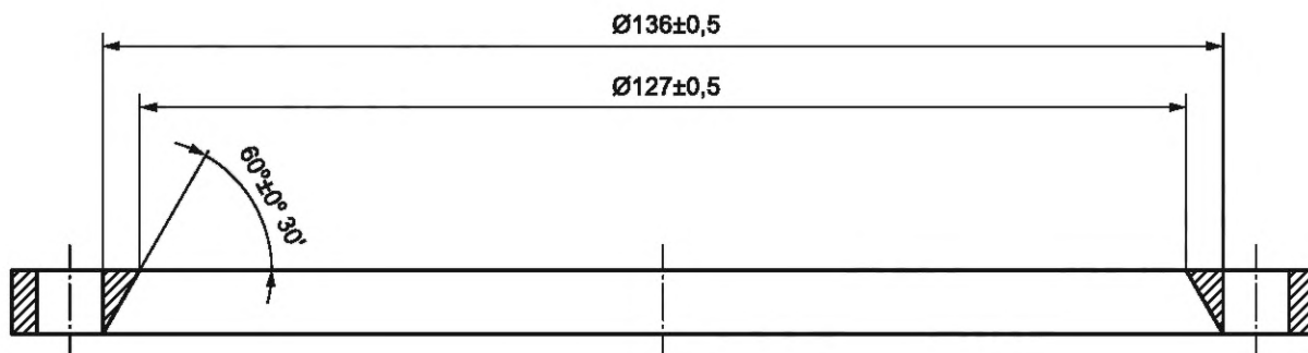
Рисунок 2 — Прижимное кольцо
