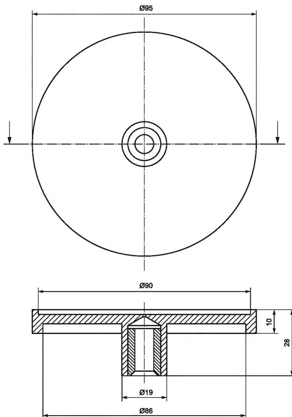
Рисунок 3 — Корпус держателя испытываемой пробы
