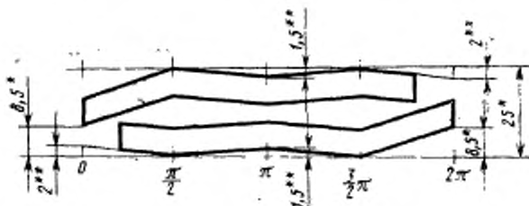
Развернутое положение для построения инструмента
