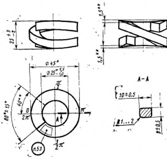
Развернутое положение для построения инструмента
