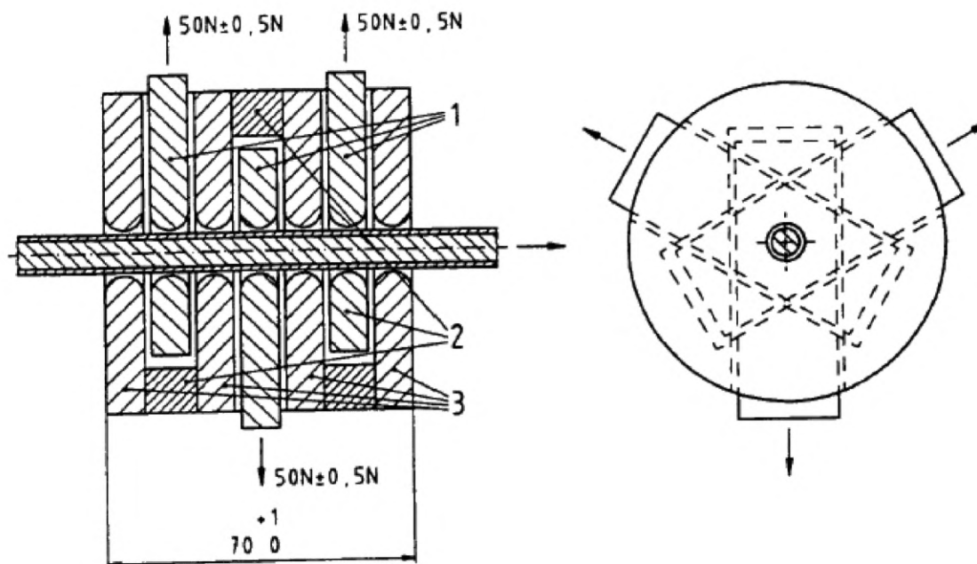
1 — движущие пластины; 2 — пространство; 3 — закрепленные пластины
