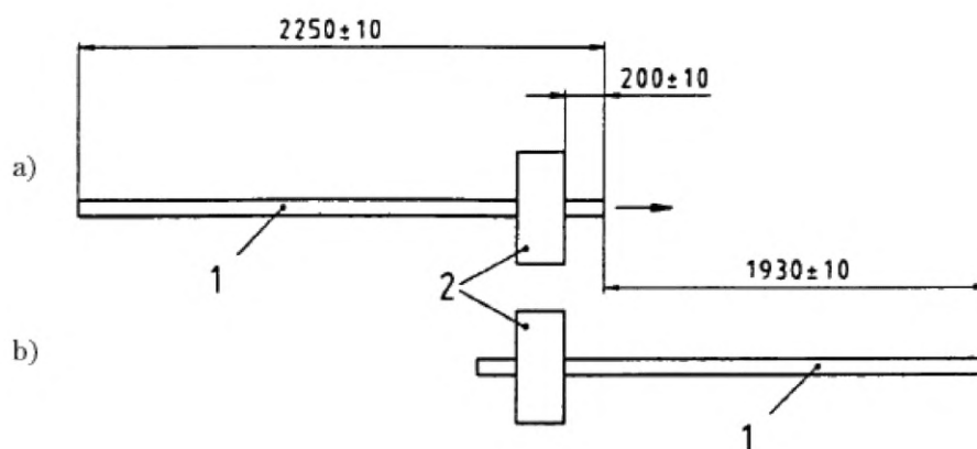
а) расположение образца до испытания; б) расположение образца после испытания; 1 — образец каната; 2 — устройство для определения смещения оболочки (см. рисунок 3)
