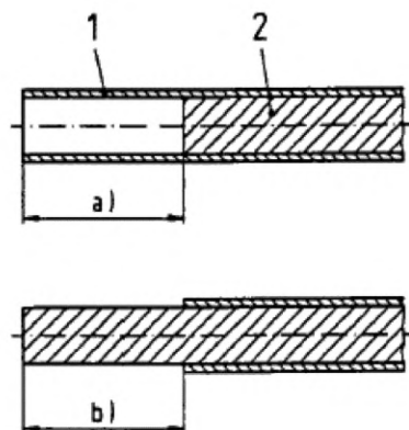
а) смещение оболочки (положительное); б) смещение оболочки (отрицательное); 1 — оболочка; 2 — сердечник
