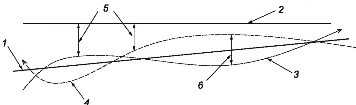
1 — линия A—B; 2 — постоянная линия на поверхности земли; 3 — предыдущая траектория перемещения репрезентативной точки машины; 4 — следующая траектория перемещения репрезентативной точки машины; 5 — относительные измерения позиции отслеживающим датчиком; 6 — относительная XTE
