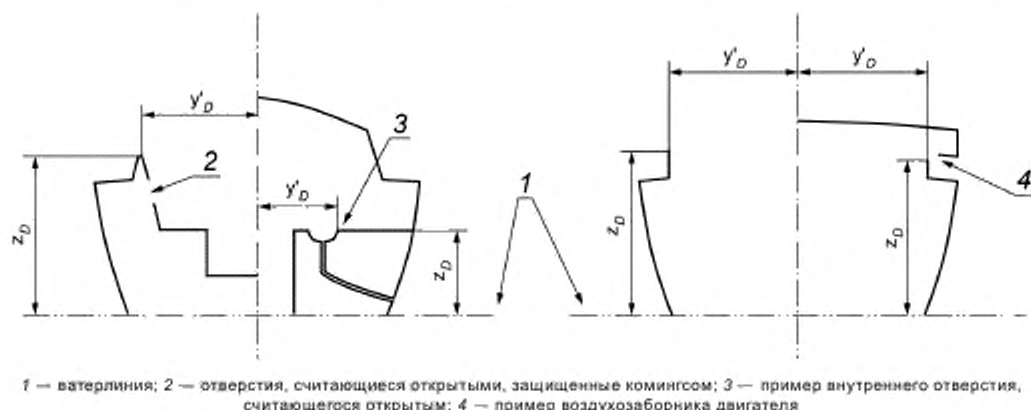
Рисунок С.1 — Приблизительный метод определения угла заливания
