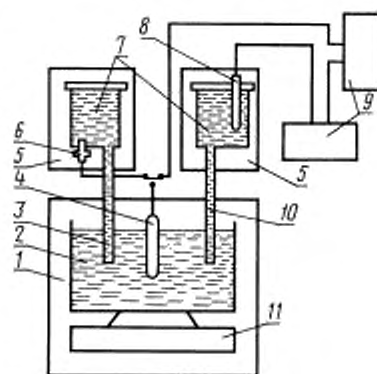
Схема установки для определения потенциала электродов
