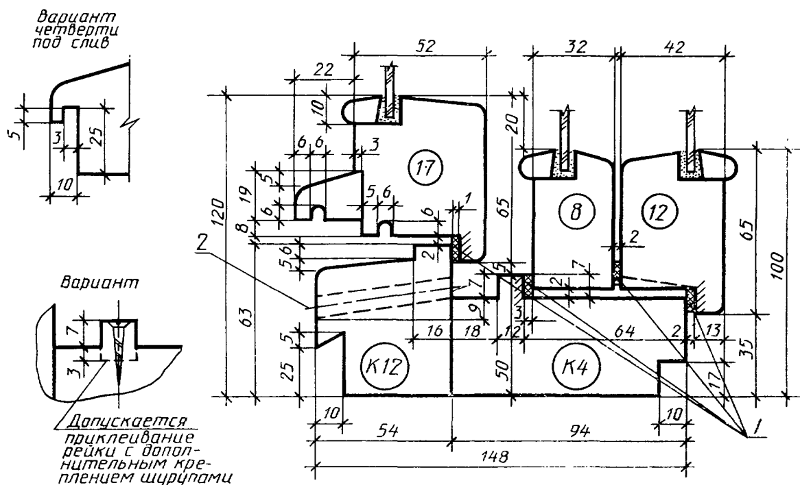
Сечение В2
