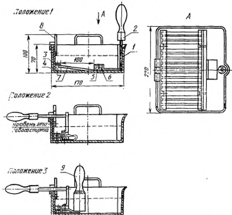
1—ванна; 2—ручка; 3—зажим 1; 4—брусек; 5—зажим 2; 6—брусек; 7—образцы; 8—защелка; 9—пестик
