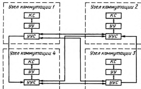
Распределенная система управления сетью связи
