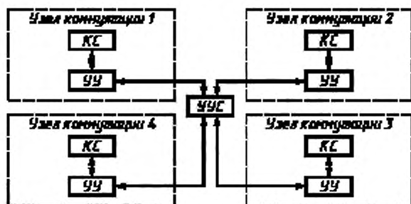
Централизованная система управления сетью связи
