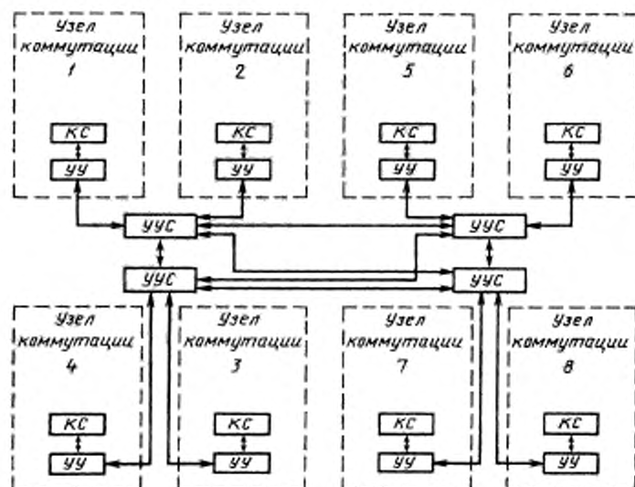
Децентрализованная система управления сетью связи
