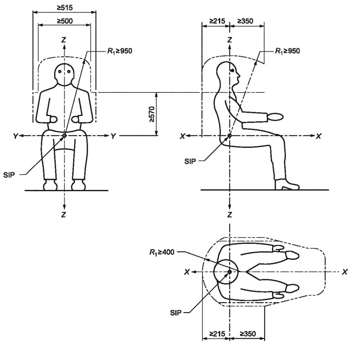
Рисунок 1 — Рабочее пространство вокруг сиденья инструктора
