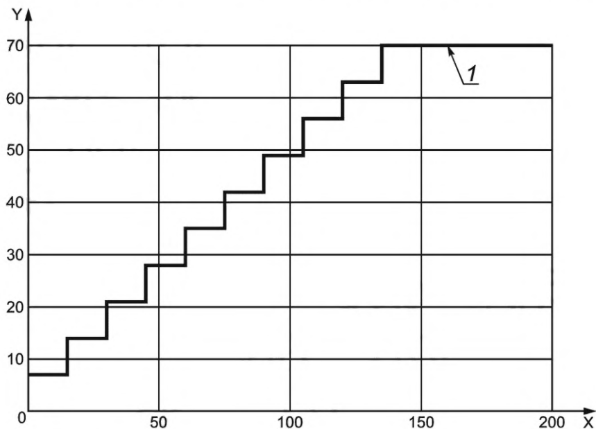
X — выдержка в минутах; Y — давление в МПа; 1 — выдержка при максимальном давлении в течение 8 ч Рисунок К.1 — График испытания уплотнительных свойств резьбовой смазки
