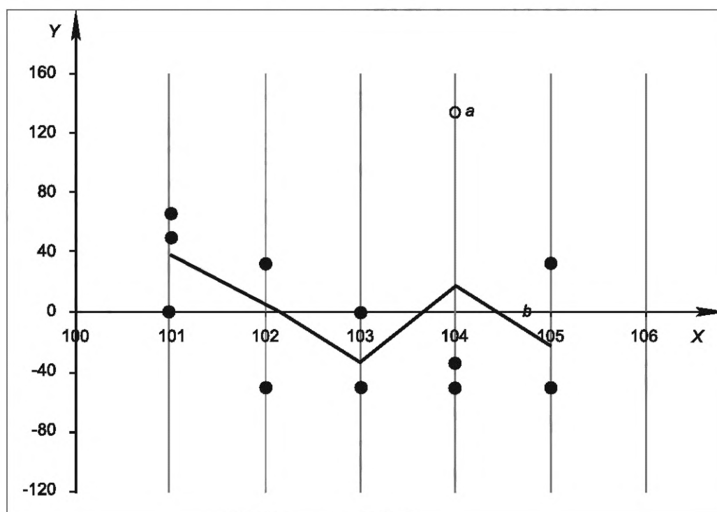
Рисунок Е.13 — Показатели функционирования для каждого тура программы проверки квалификации (данные таблицы Е.12)
