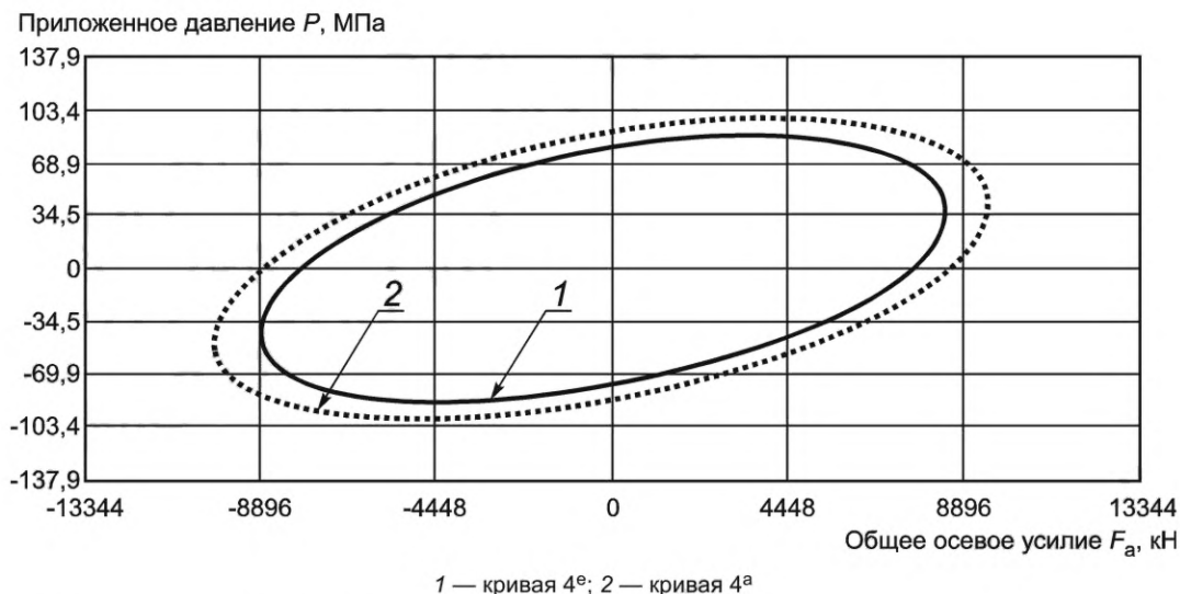
Рисунок D.12 — Кривые фактического VME испытательного образца тела трубы при температуре окружающей среды (4 а ) и при повышенной температуре (4 е )
