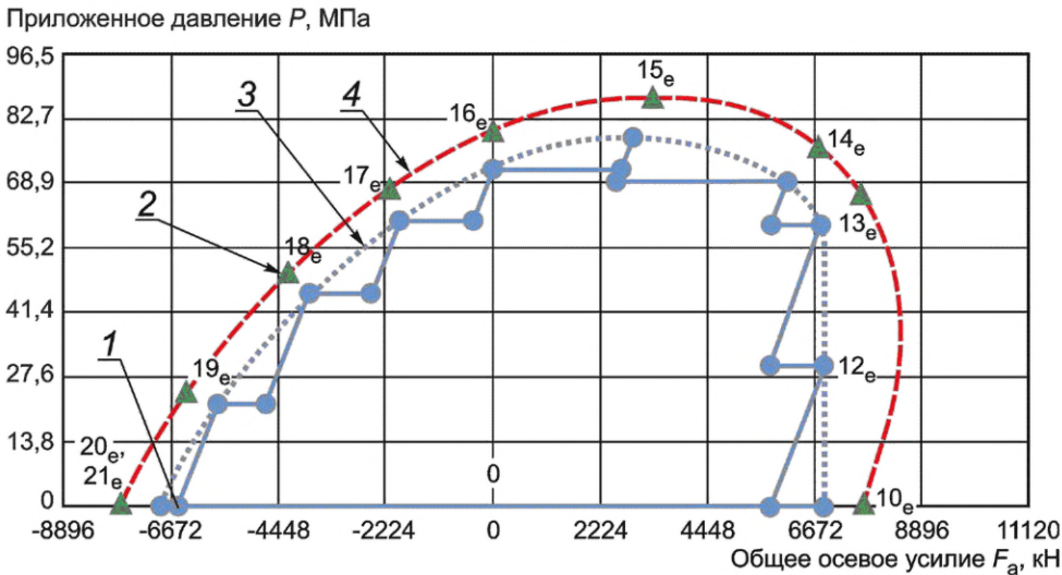
Рисунок D.26 — A e 90 % (QI, QII), TS-A этапы нагрузки 1—24
