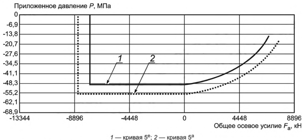
Рисунок D.13 — Кривые фактического давления смятия по API испытательного образца тела трубы при температуре окружающей среды 5 а и при повышенной температуре 5 е
