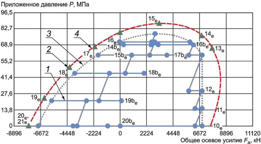
Рисунок D.22 — B e b 90 % (QI, QII, QI), TS-B этапы нагрузки 67—155
