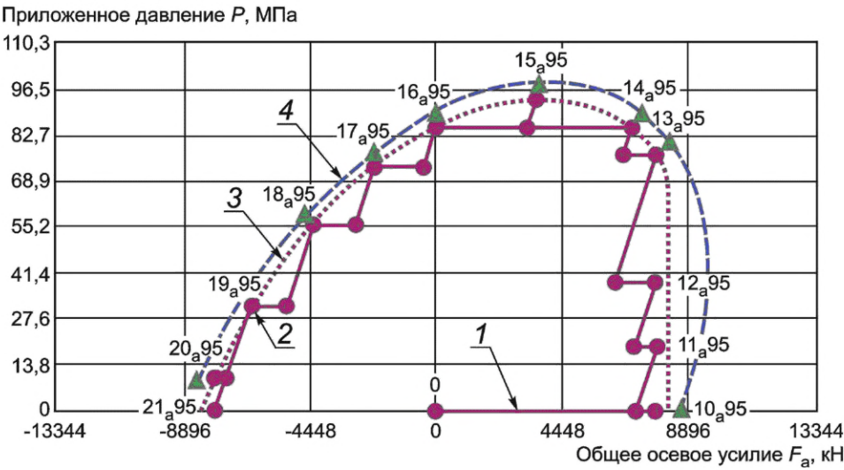
1 — точки TLE a 95; 2 — точки CEE a ; 3 — 95 % CEE a ; 4 — кривая 4 a Рисунок D.21 — B a 95 % (QI, QII, QI), TS-B этапы нагрузки 20—66
