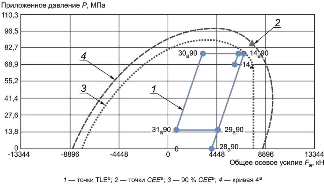
Рисунок D.25 — Пять механических циклов, TS-C этапы нагрузки 45—69
