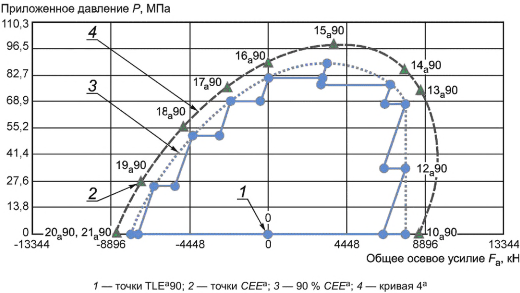
Рисунок D.32 — A a 90 % (QI, QII), TS-A этапы нагрузки 176—198
