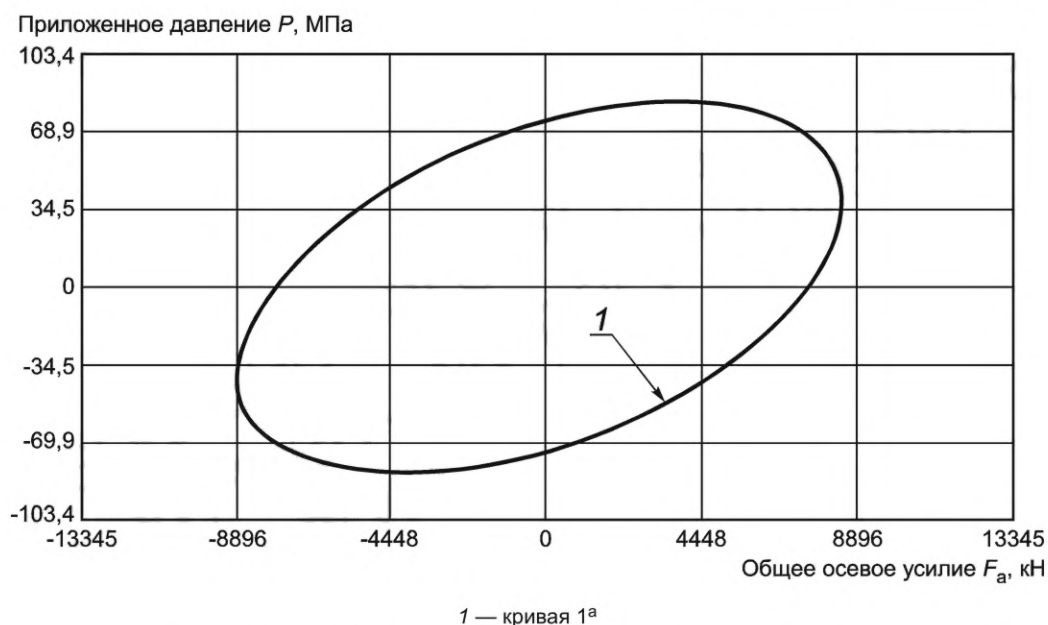
Рисунок D.4 — Кривая 1 a номинального VME тела трубы при температуре окружающей среды
