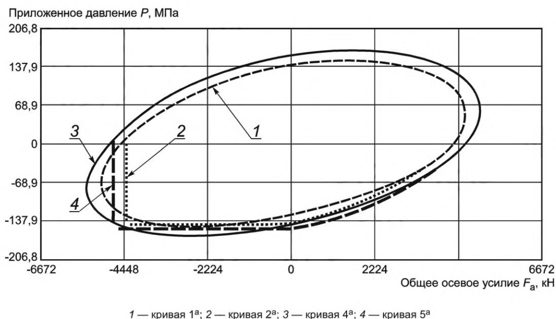
Рисунок D.36 — Эталонные кривые испытательного образца тела трубы (кривые 1 a , 2 a , 4 a и 5 a )
