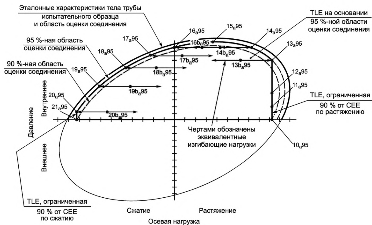
Рисунок 30 — Пример точек нагрузки TS-B при температуре окружающей среды с изгибом при величине нагрузки 95 % от СЕЕ при совпадении эталонных характеристик тела трубы и области оценки резьбового соединения с ограничением растяжения и сжатия до 90 % от СЕЕ
