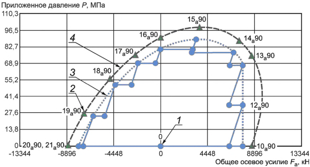
1 — точки TLE a 90; 2 — точки CEE a ; 3 — 90 % CEE a ; 4 — кривая 4 a
