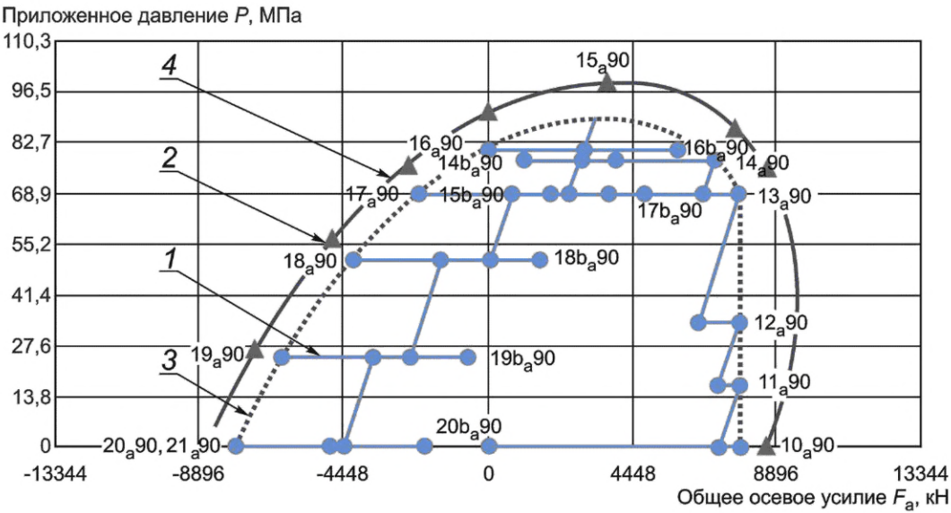
1 — точки TLE a 90; 2 — точки CEE a ; 3 — 90 % CEE a ; 4 — кривая 4 a Рисунок D.23 — B^a_b 90 % (QI, QII, QI), TS-B этапы нагрузки 156—244
