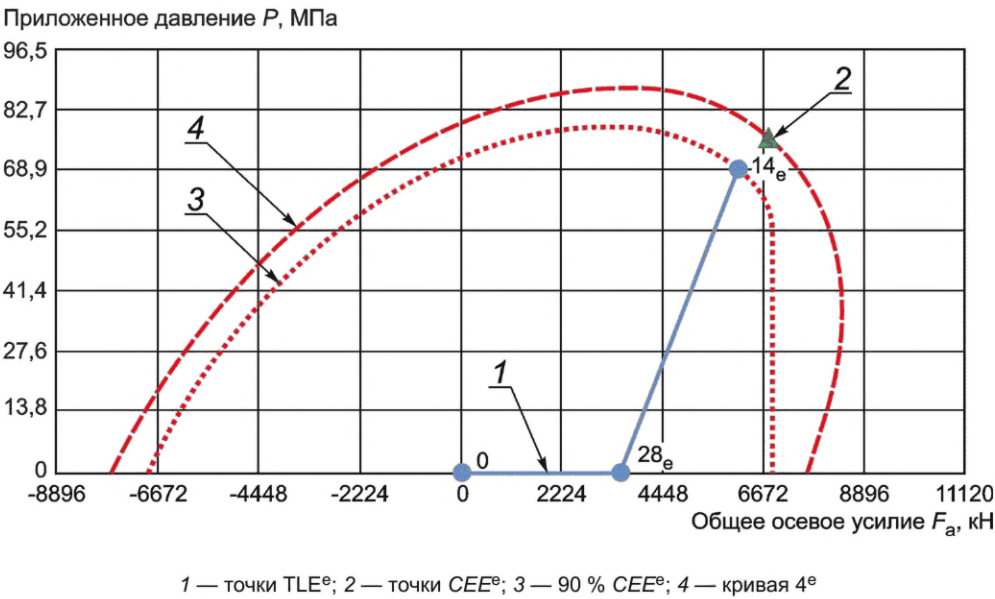
Рисунок D.24 — Десять термических циклов, TS-C этапы нагрузки 1—44
