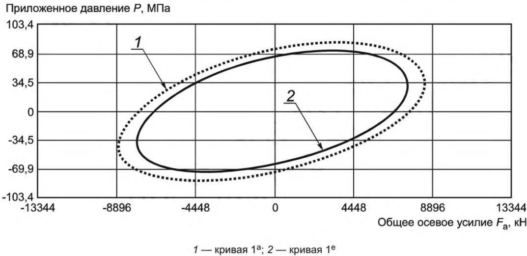
Рисунок D.9 — Кривые номинального VME испытательного образца тела трубы при температуре окружающей среды (1 a ) и при повышенной температуре (1 e )
