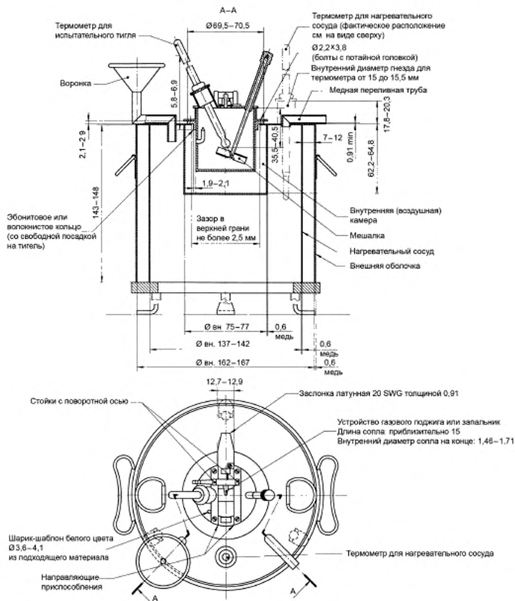
Рисунок А.2 — Прибор для определения температуры вспышки по Абелью в сборе
