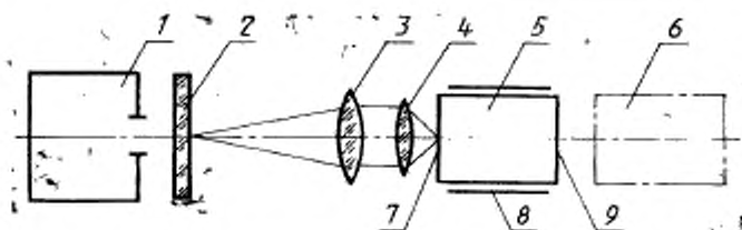
1—осветитель; 2—сетка; 3—коллимационный объектив; 4—проекционный объектив; 5—ЭОП; 6—яркомер; 7—фотокатод; 8—светонепроницаемая камера; 9—экран
