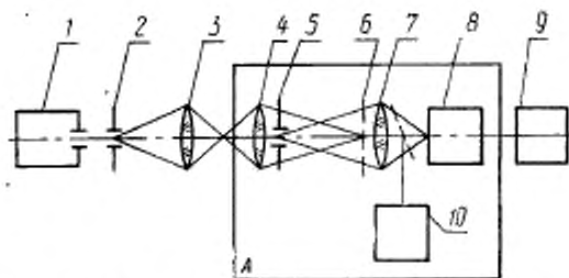
1 — осветитель; 2 — диафрагма со щелью; 3 — входная оптика (микрообъектив в обратном ходе); 4 — выходной микрообъектив; 5 — выходной эррочок микрообъектива; 6 — анализирующий растр; 7 — коллектив; 8 — приемник излучения; 9 — регистрирующее устройство; 10 — микроскоп; А — анализирующий блок
