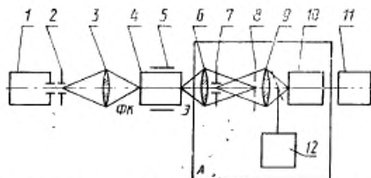
1 — осветитель; 2 — диафрагма со щелью; 3 — входная оптика (микрообъектив в обратном ходе); 4 — ЭОП; 5 — держатель ЭОП; 6 — выходной объектив микрообъектива; 7 — выходной экран микрообъектива; 8 — анализирующий растр; 9 — коллектив; 10 — приемник излучения; 11 — регистрирующее устройство; 12 — микроскоп; ФК — фотокатод; Э — экран; А — анализирующий блок
