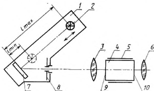
1—осветитель; 2—лампа накаливания; 3—объектив; 4—ЭОП; 5—держатель ЭОП; 6—окулярная оптика; 7—пластина диффузного рассеивания; 8—диафрагма с калиброванным отверстием; 9—Фотокатод; 10—экран
