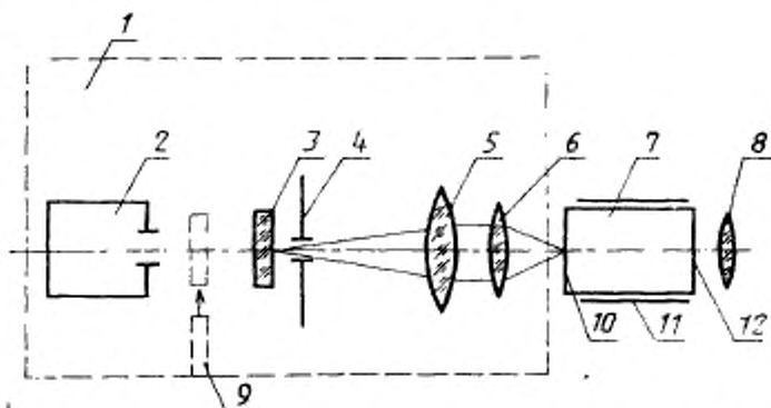
1—проектор; 2—осветитель; 3—мира; 4—диафрагма с окном; 5—коллимационный объектив; 6—проекционный объектив; 7—ЭОП; 8—окулярная оптика; 9—светофильтр; 10—фотокатод; 11—держатель ЭОП; 12—экран
