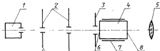
1—источник света; 2—светозащитная диафрагма; 3—диафрагма с калиброванным отверстием или сетка; 4—ЭОП; 5—окулярная оптика; 6—фотокатод; 7—держатель ЭОП; 8—экран
