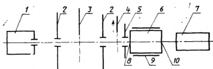
1—источник света; 2—светозащитная диафрагма; 3—заслонка; 4—непрозрачный диск; 5—диафрагма; 6—ЭОП; 7—яркомер; 8—фотокатод; 9—держатель ЭОП; 10—экран
