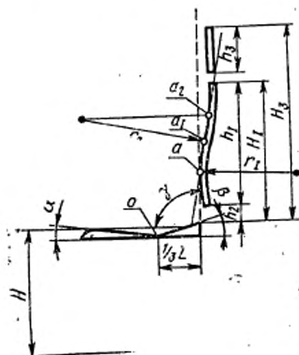
Кресло с профилированными элементами
