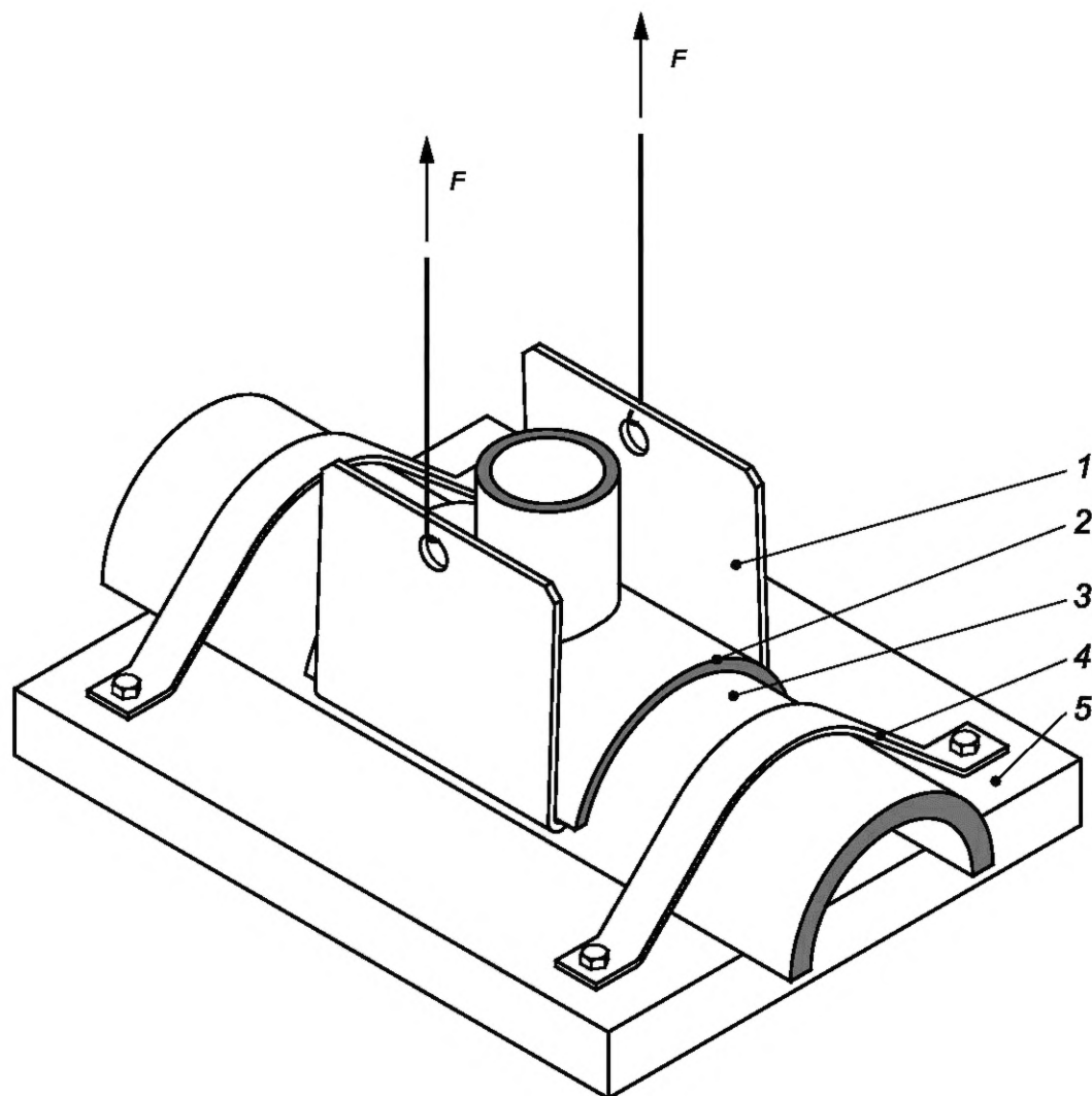
1 — зажимное устройство; 2 — седловой отвод из ПЭ; 3 — труба из ПЭ; 4 — зажим; 5 — опорная плита; F — усилие отслаивания
