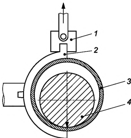
1 — зажимное устройство, обеспечивающее вращение образца относительно точки приложения нагрузки; 2 — седловый отвод из ПЭ; 3 — труба из ПЭ; 4 — нагружающий штифт
