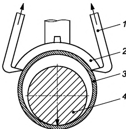
1 — зажимное устройство; 2 — седловый отвод из ПЭ; 3 — труба из ПЭ; 4 — нагружающий штифт
