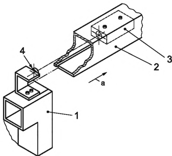
б) Низкоуровневое кодированное блокировочное устройство Типа 3 или 4
