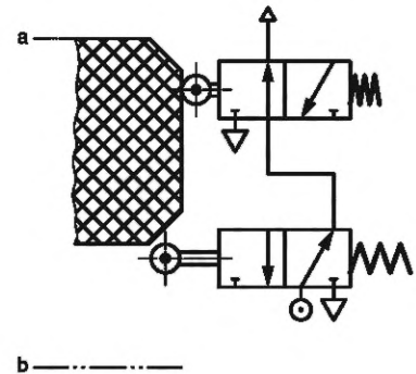
Рисунок А.4 — Одиночный клапан (выходная система) с прямым механическим действием одиночного клапана подвижным ограждением
