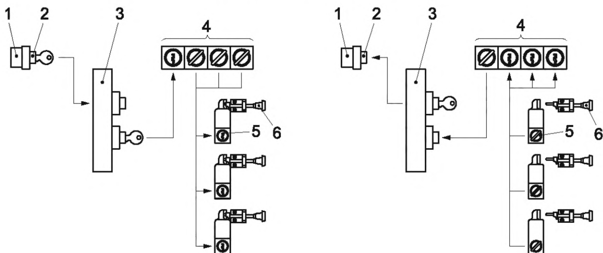
Рисунок В.5 — Простая базовая система
