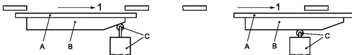
а) Подвижное ограждение закрыто
