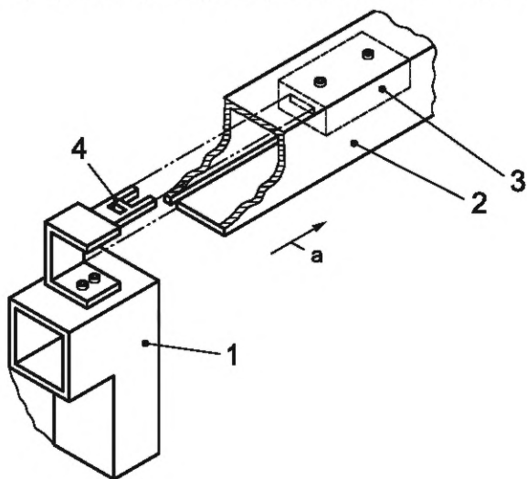
а) Блокировочное устройство Типа 2
