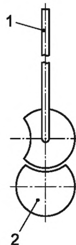
б) Подвижное ограждение не закрыто
