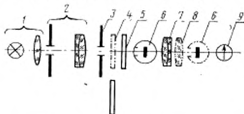
1 — осветитель; 2 — коллиматор; 3 — ирисовая диафрагма; 4 — непрозрачный экран; 5 — светофильтр; 6 — фотоприемник; 7 — испытуемый объектив; 8 — вспомогательная оптическая система; 9 — измерительный прибор
