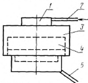
1—брызгало гидроциклонное; 2—штуцер для подачи промывочной воды; 3—корпус приставки; 4—сито; 5—патрубок для вывода под решетчатого продукта
