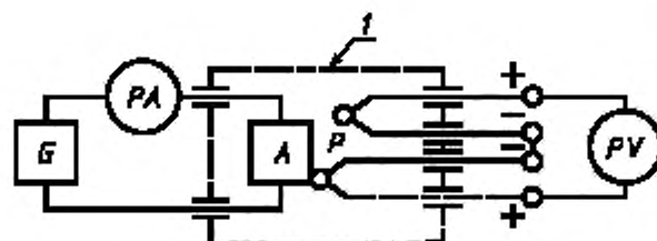
Г — стабилизированный источник тока; РА — измеритель тока; А — изделие; I — испытательная камера; Р — измеритель температуры; РУ — милливольтметр
