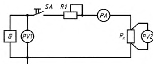
G — источник тока; SA — выключатель; R1 — переменный резистор; PA — амперметр; PV1 , PV2 — вольтметры, R_x — сопротивление измеряемого контакта
