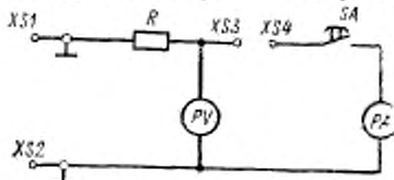
РА—амперметр; PV—вольтметр.
