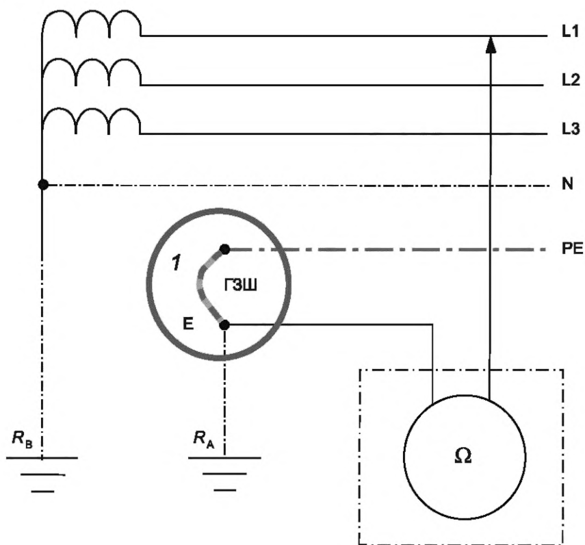
1 — заземляющий проводник, временно отключенный от главной заземляющей шины (ГЗШ)
