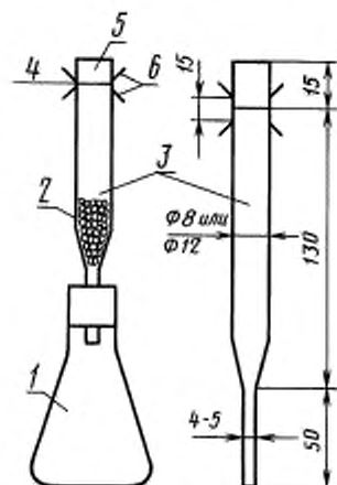
Прибор для определения мышьяка визуально-колориметрическим методом
