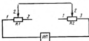
R1 и R2 — проверяемые резисторы; ИП — источник питания постоянного или переменного тока
