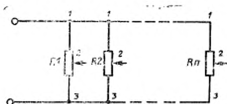
R_1 , R_2 , R_n — испытываемые резисторы, 1, 3 — неподвижные контакты; 2 — подвижный контакт
