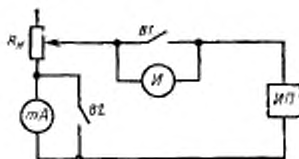
В1—испытываемый выключатель; В2—выключатель для защиты амперметра; И—индикатор; ИП—источник питания постоянного или переменного тока; мА—миллиамперметр; R_n —нагрузочный резистор
