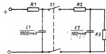
S1 —испытываемый выключатель; R1 , R2 , R3 —резисторы заданного режима, C —конденсаторы заданного режима
