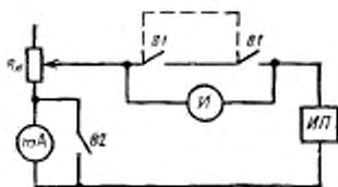
В1—испытываемый выключатель; В2—выключатель для защиты амперметра; И—индикатор; ИП—источник питания постоянного или переменного тока; мА—миллиамперметр; R_n —нагрузочный резистор
