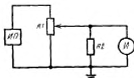
R1 —проверяемый резистор; R2 —нагрузочный резистор; И —индикатор; ИП —источник питания постоянного или переменного тока
