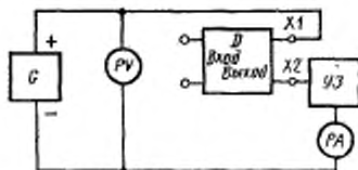
G —генератор постоянного тока; PV —измеритель напряжения; D —измеряемый прибор; X1 , X2 —контакты подключения измеряемого прибора; UZ —устройство защиты измеряемого прибора от перегрузки при коротком замыкании; PA —измеритель тока
