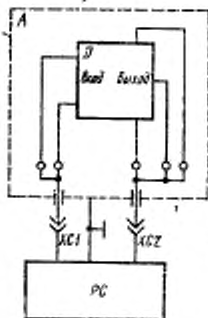
А—устройство подключения; D—измеряемый прибор; ХС1, ХС2—разъемное соединение устройства подключения и измерителя емкости; PC—измеритель емкости
