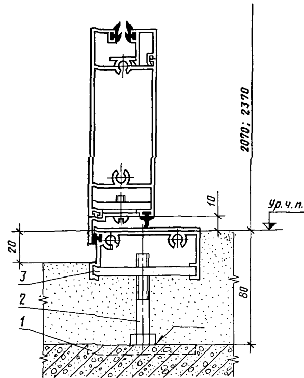
Сечение 2 Дверь с порогом
