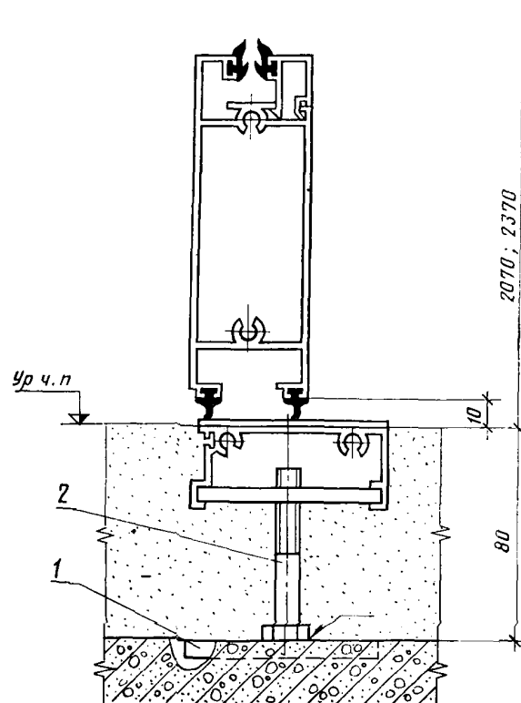
Сечение 2 Дверь без порога
