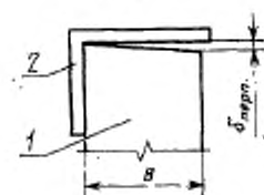
Схема определения перпендикулярности сторон
