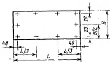
Схема расположения точек измерения толщины панели
