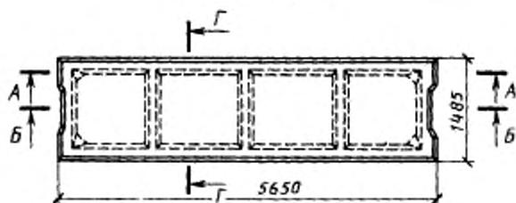
Плита типоразмера П2
