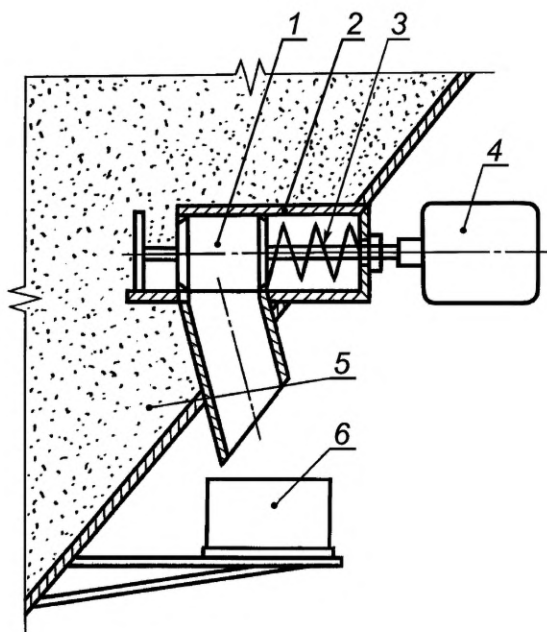
1 — дозатор; 2 — корпус; 3 — пружина; 4 — электромагнит; 5 — бункер; 6 — емкость для пробы
