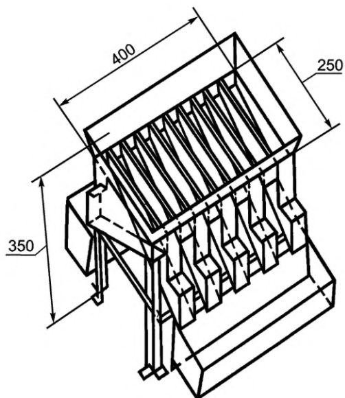
Рисунок 9 — Делитель Джонса
