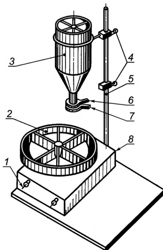
1 — включатель; 2 — делитель; 3 — усреднитель; 4 — держатель; 5 — штанга; 6 — отсекающий; 7 — диафрагма; 8 — электродвигатель
