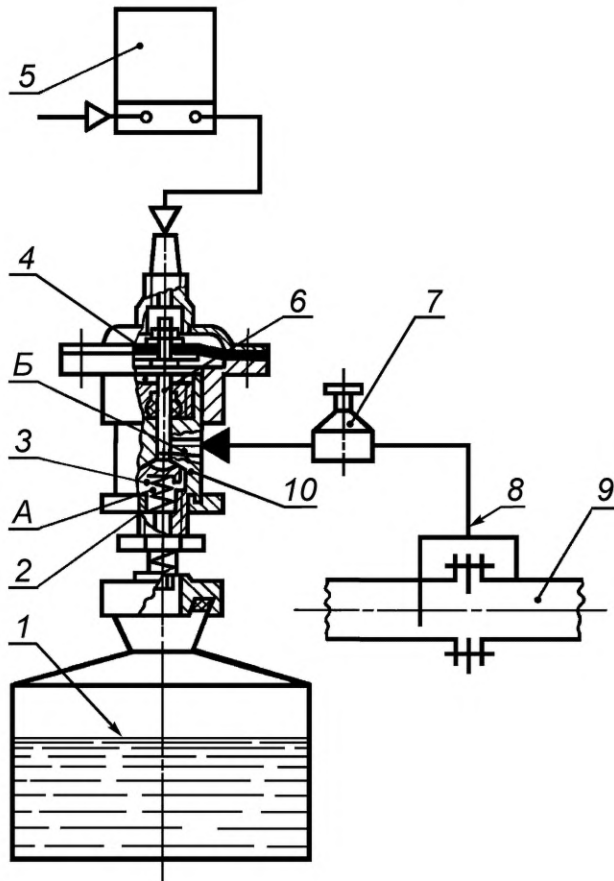
Рисунок 1 — Автоматический пробоотборник типа АП-2М1 для жидких продуктов
