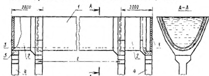
Схема гидростатических испытаний лотка на водонепроницаемость
