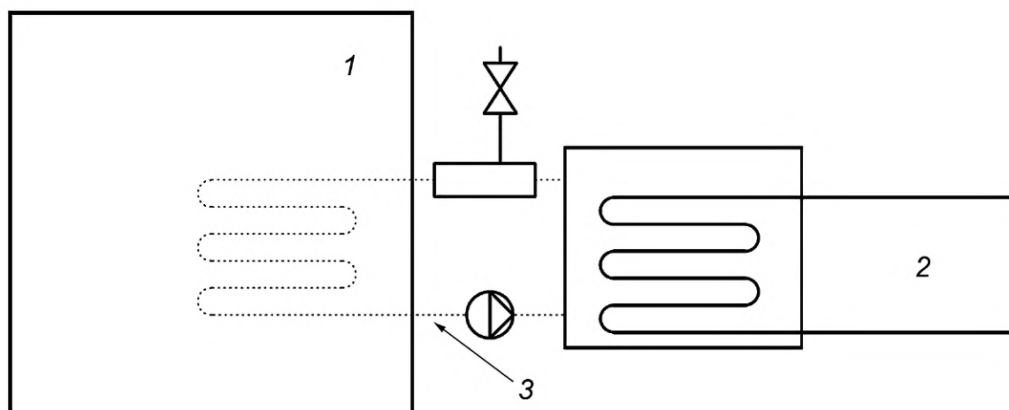
Рисунок 7 — Закрытая промежуточная система с вытяжкой
