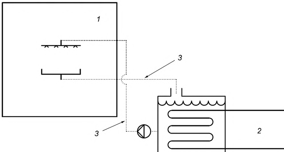
Рисунок 4 — Открытая оросительная система с открытым уровнем
