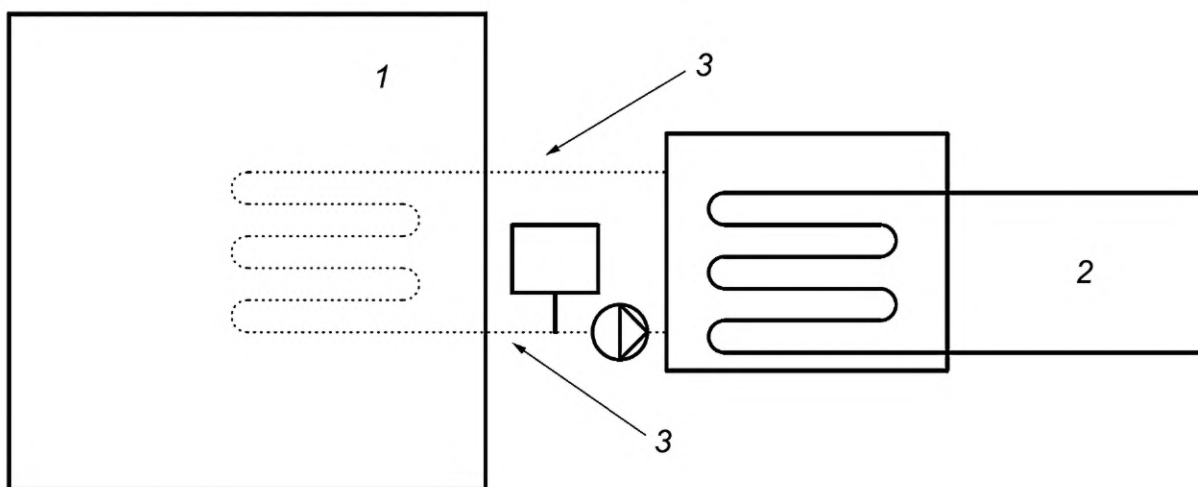
Рисунок 5 — Закрытая промежуточная система
