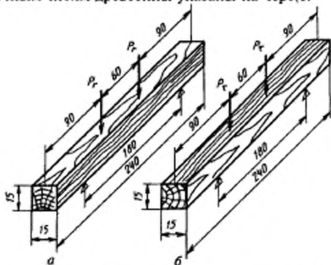
a — нагрузка, изгибающая образец в радиальном направлении ( P_r ); б — нагрузка, изгибающая образец в тангенциальном направлении ( P_t ).
