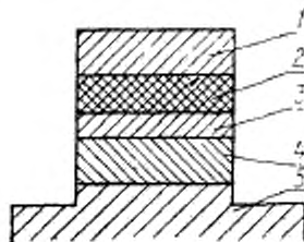
1 — тонкий стержень; 2 — образец испытуемый; 3 — контактная пластина; 4 — пластина; 5 — основание
