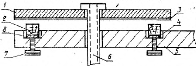
1—шлифовальный диск; 2—образец; 3—шлифовальная шкурка; 4—подкладка; 5—рычаг; 6—полюс вал; 7—винт; 8—зажимная рамка
